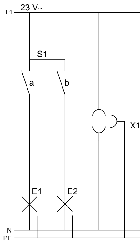
Stroomkringschema
